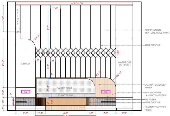
ELEVATION-A
